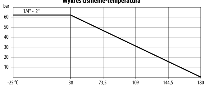
Wykres ciśnienie-temperatura
