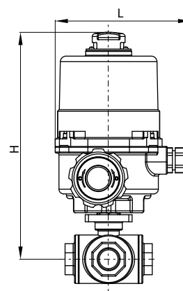
TYP BV531 - Z NAPĘDEM ELEKTRYCZNYM ON-OFF
