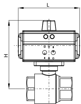
TYP BV201 - Z NAPĘDEM PNEUMATYCZNYM
