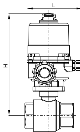
TYP BV201 - Z NAPĘDEM ELEKTRYCZNYM ON-OFF
